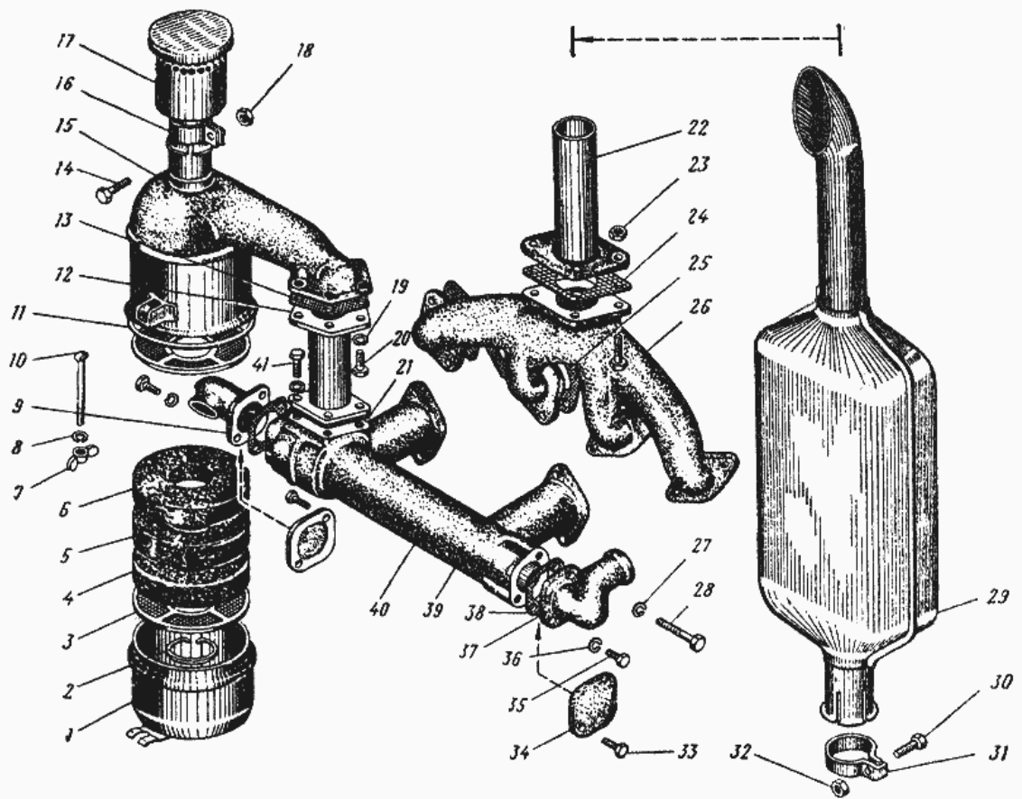
Рис. 19. Газопровод, воздушный фильтр, глушитель
